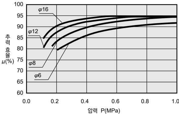
[그림2] 추력 효율 - 압력의 관계
